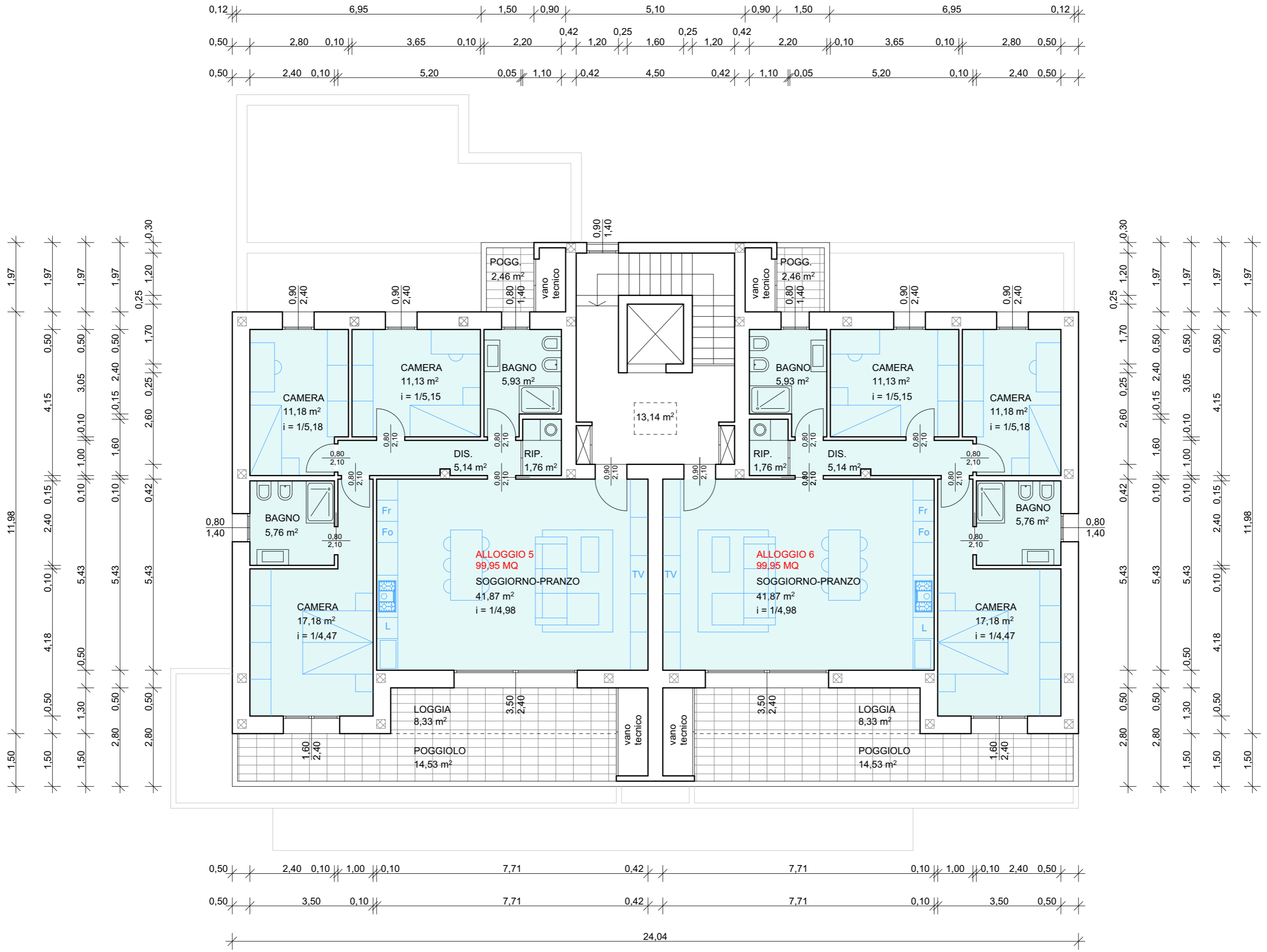
PIANTA PIANO SECONDO Scala 1:100
